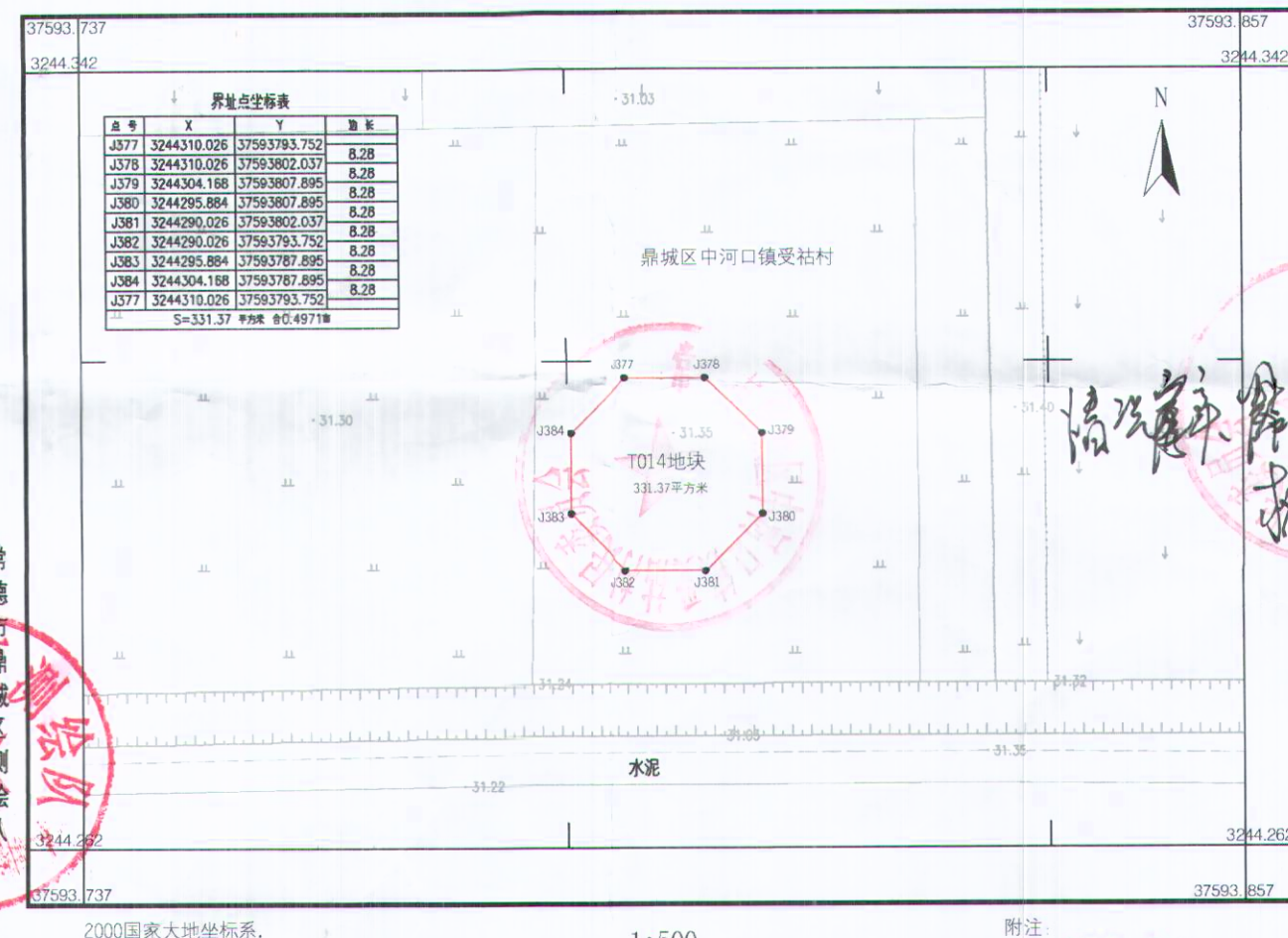
鼎城区200MW风电场项目T014地块勘测定界图 344.82-356.77
