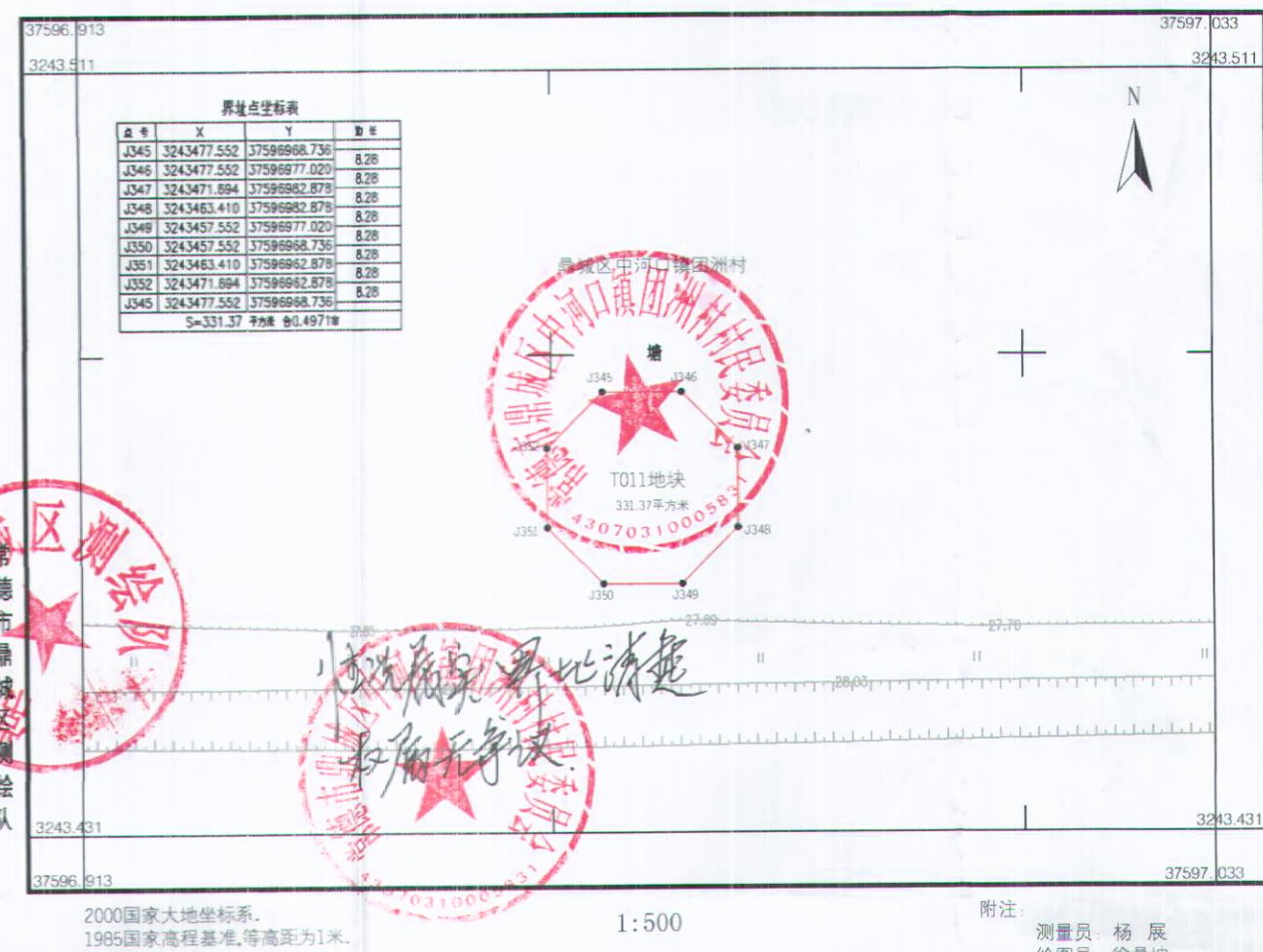
鼎城区200MW风电场项目T011地块勘测定界图 343.41-356.93
