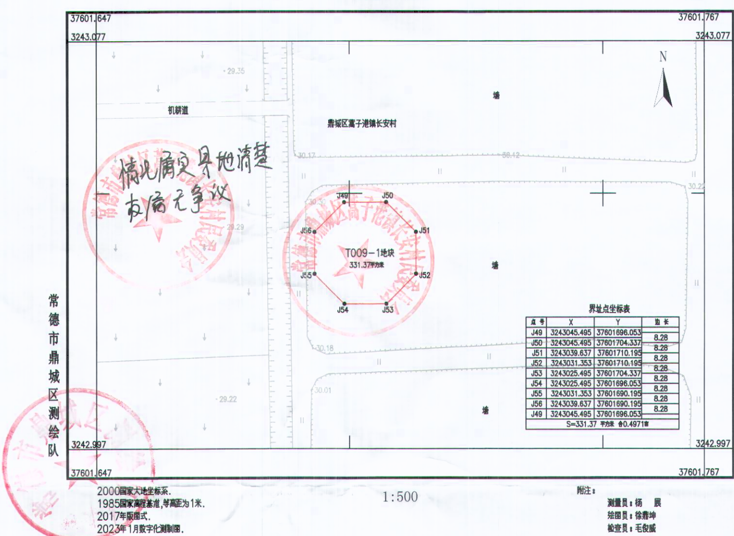
鼎城区200MW风电项目T009-1地块勘测定界图
