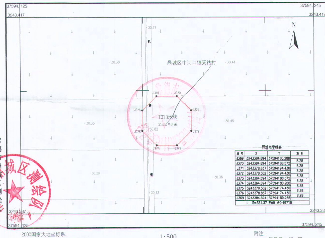
鼎城区200MW风电场项目T013地块勘测定界图 343.37-356.15
