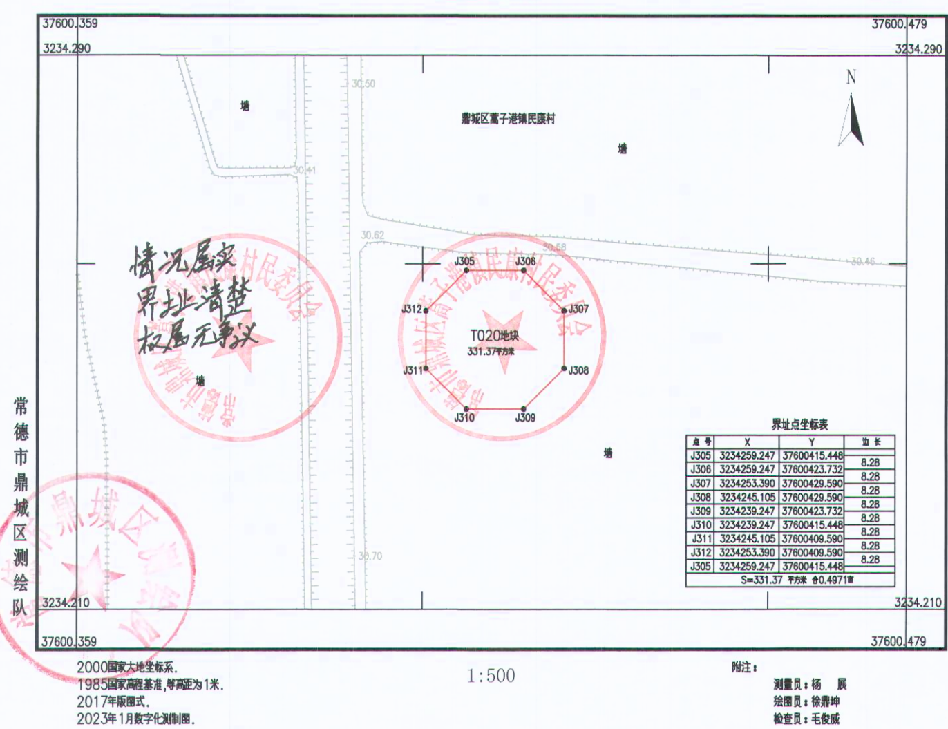
鼎城区200MW风电项目T020地块勘测定界图
