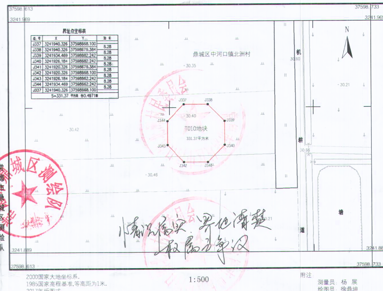
鼎城区200MW风电场项目T010地块勘测定界图 343.37-356.63
