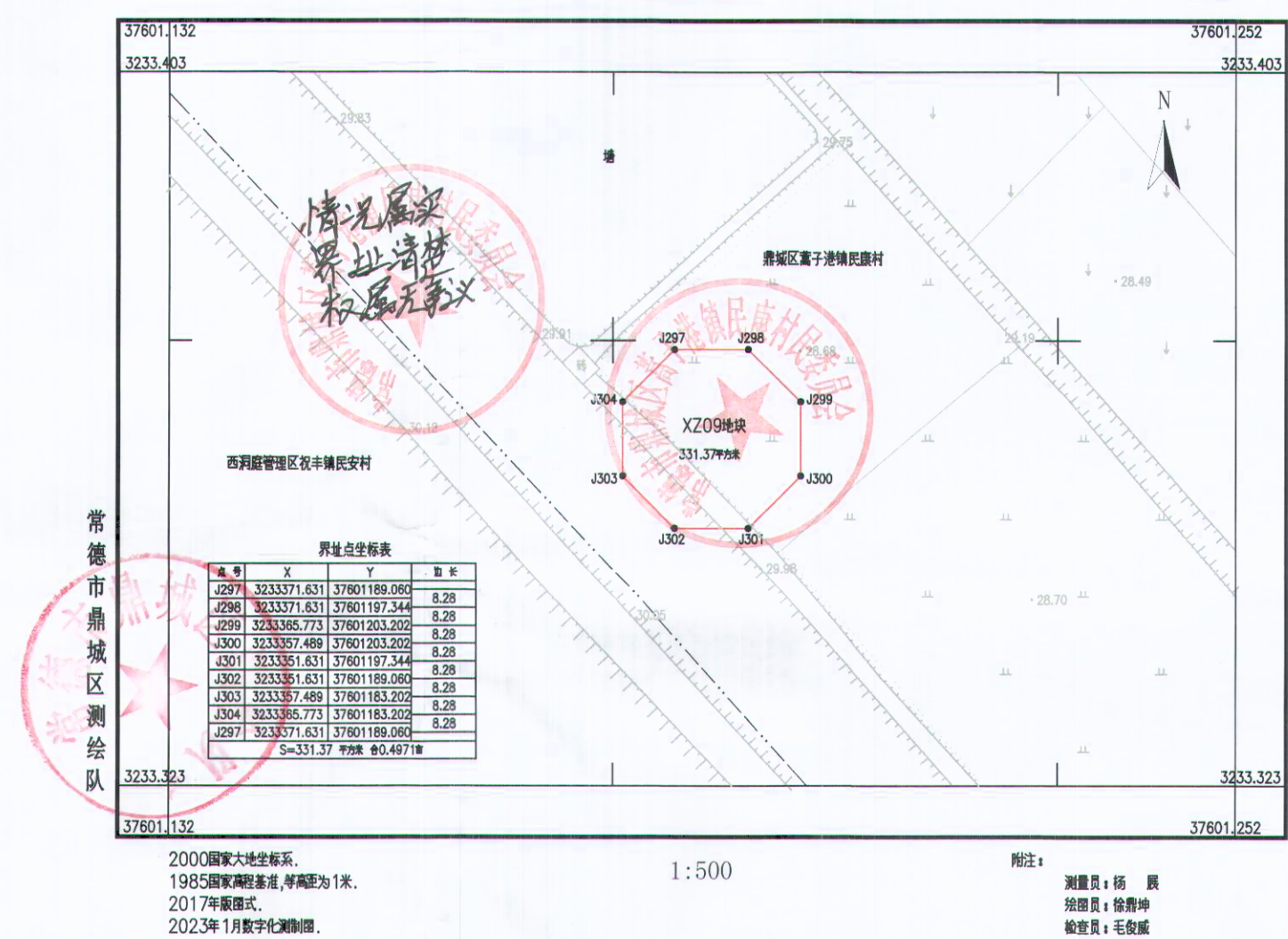
鼎城区200MW风电项目XZ09地块勘测定界图
