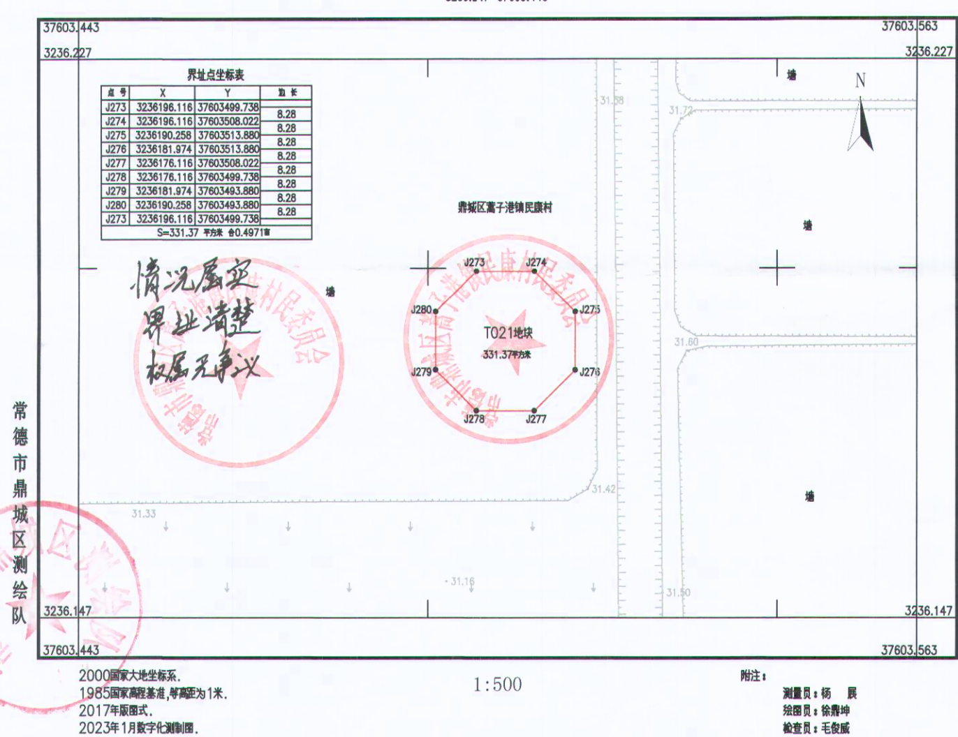
鼎城区200MW风电项目T021地块勘测定界图
