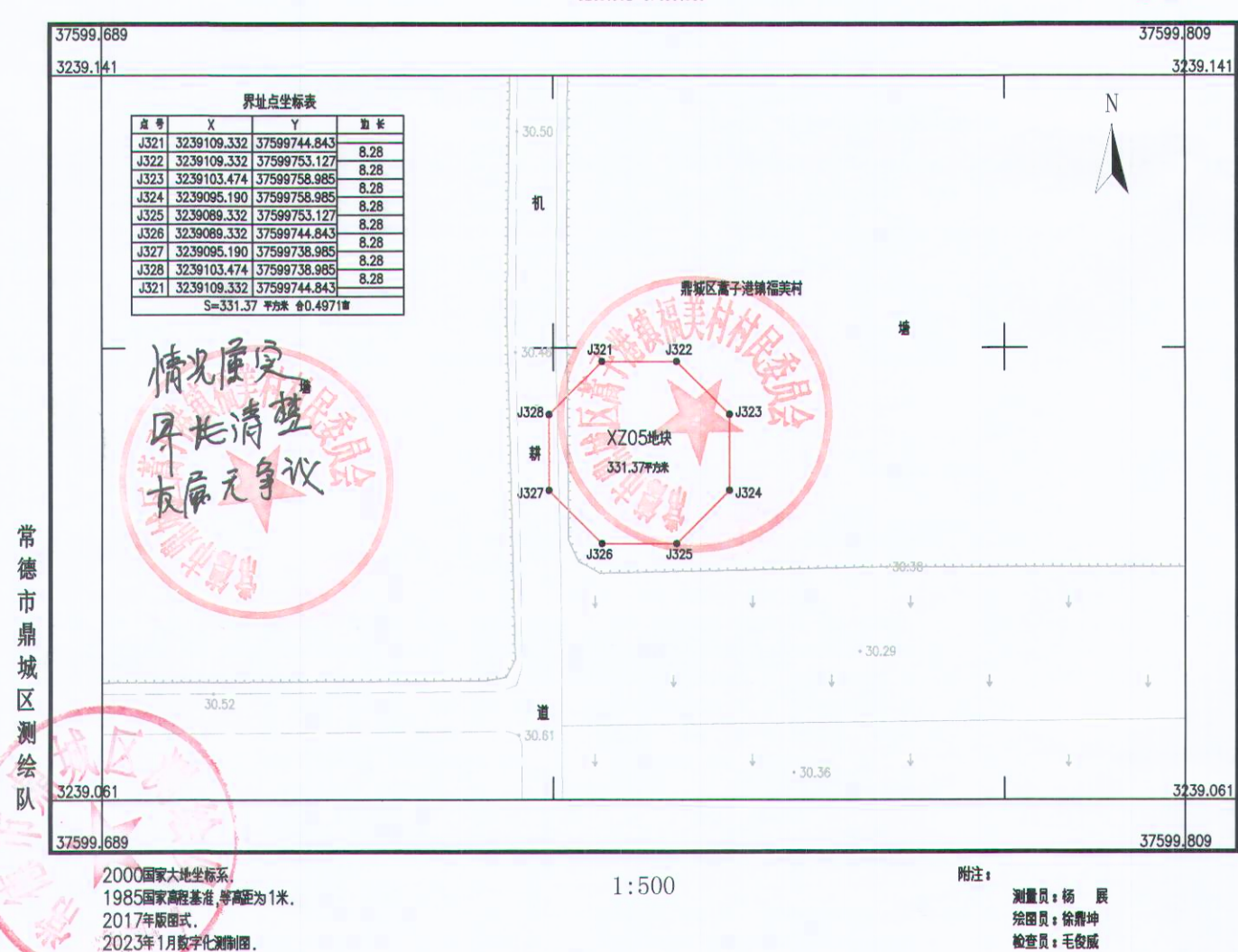
鼎城区200MW风电项目XZ05地块勘测定界图
