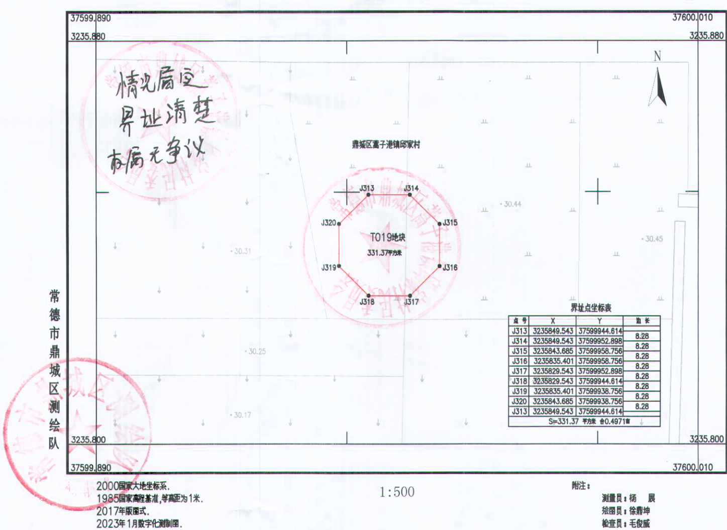
鼎城区200MW风电项目T019地块勘测定界图
