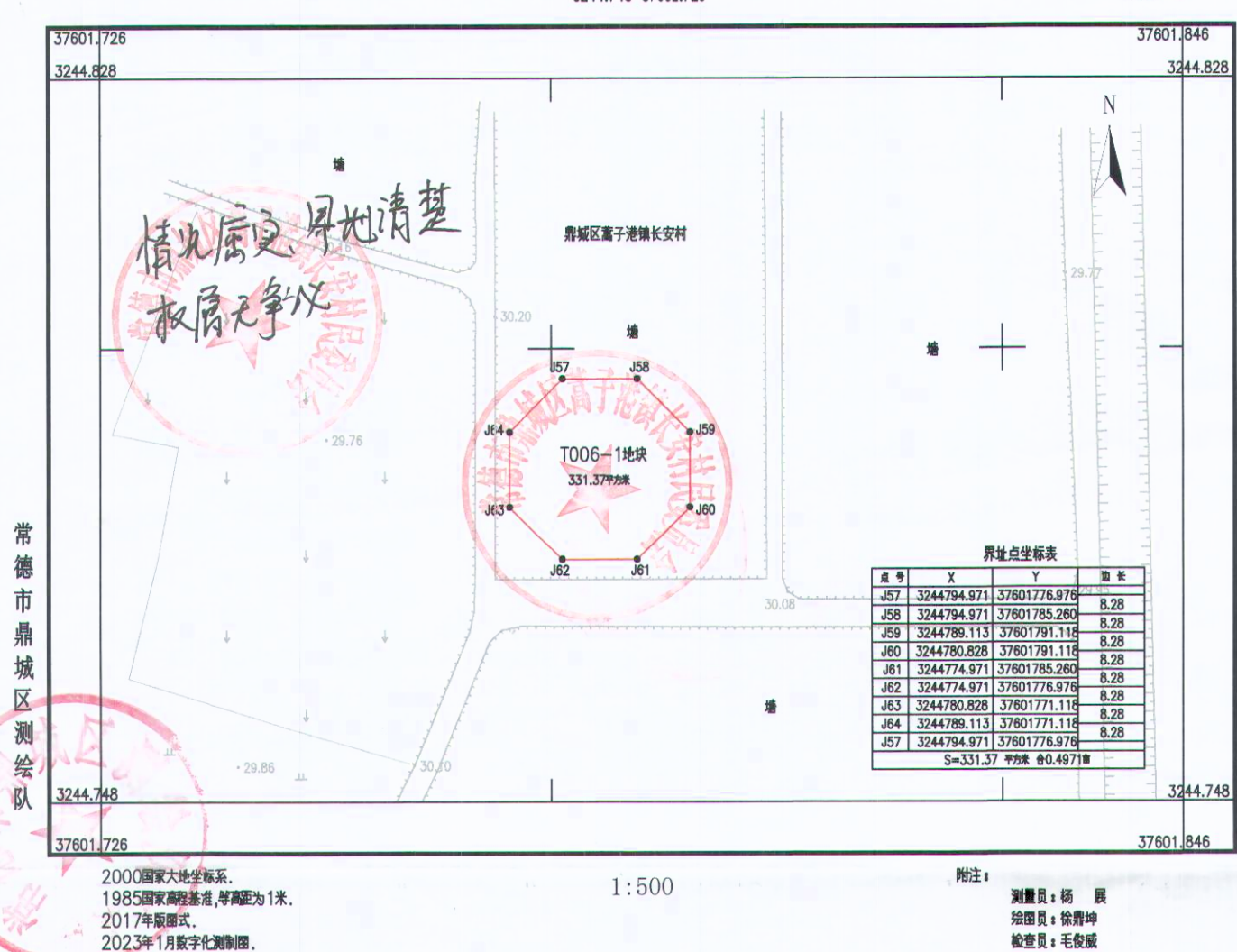
鼎城区200MW风电项目T006-1地块勘测定界图
