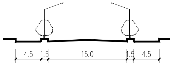
A-A断面图
